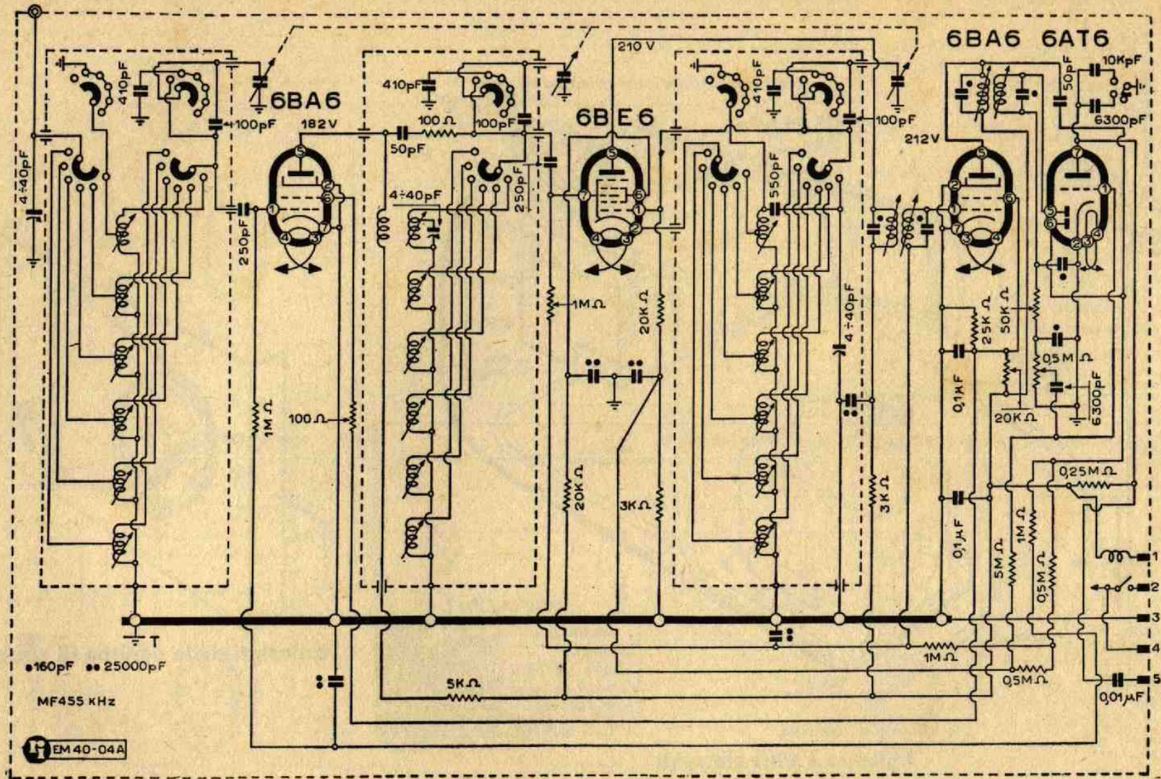
Lo schema elettrico dell'Autovox Mod. "RA 7/F., (sezione α)
